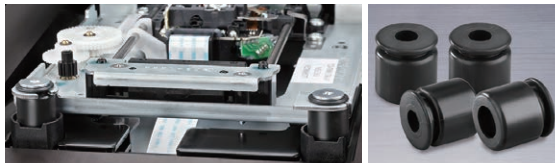
Auf Viskosedämpfern gelagerter Traverse-Mechanismus
