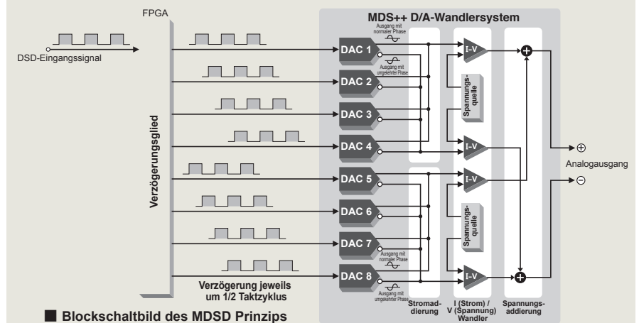
Blackschaltbild des MDSD Prinzips
