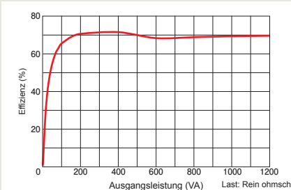
Verhältnis Ausgangsleistung/Effizienz
