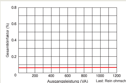
Ausgangsleistung – Gesamtklirrfaktor
