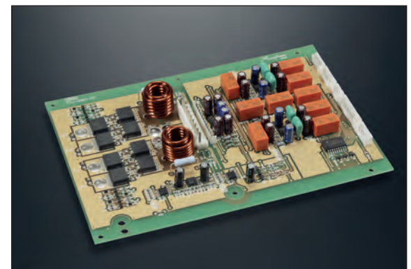
In der Endstufe setzt Accuphase erstmal auf Mosfets (links im Bild) als Schaltelemente für die Schutzschaltung
