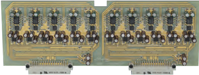
Diese Platine bildet die Lautstärkeregelung nach dem AAVA-Prinzip für einen Kanal
