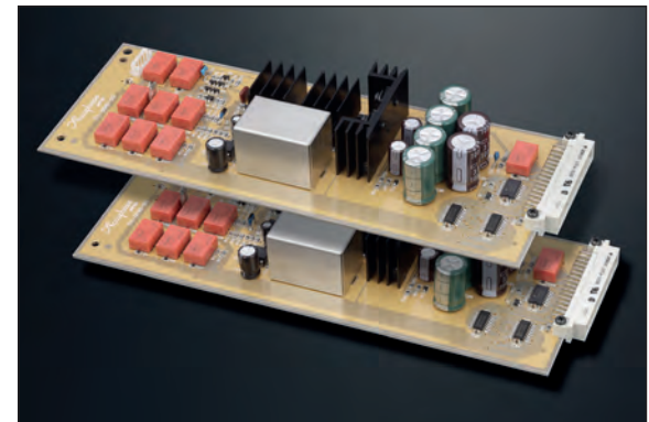
Das Phonomodul ist weitgehend diskret und sauber kanalgetrennt aufgebaut
