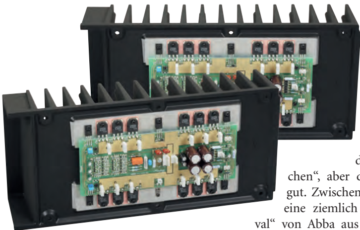
Auf den Endstufenmodulen sorgen pro Kanal zwölf Mosfets für reichlich Class-A-Leistung
